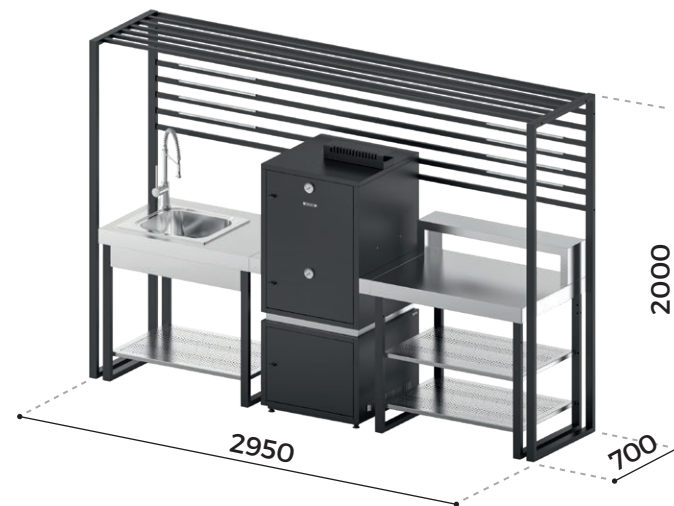
CUISINE D'EXTÉRIEUR AVEC DISPOSITIF DE FUMAGE
