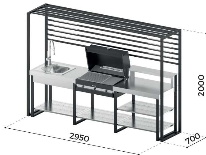
CUISINE D'EXTÉRIEUR AVEC GAZ
